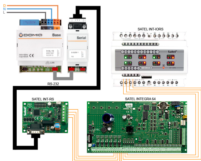
Rys 12.1: Schemat połączenia urządzeń DOMIQ i Satel
